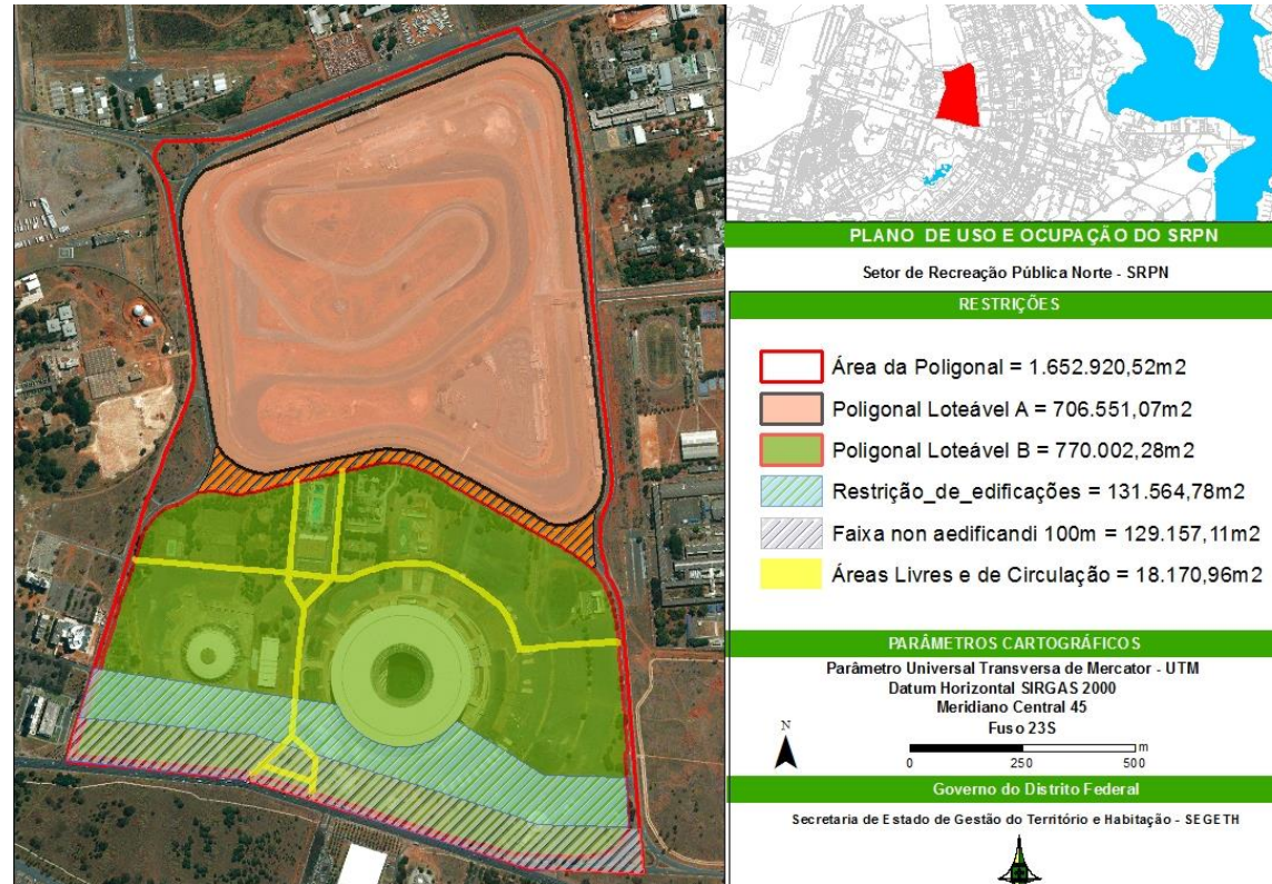
Figura 11 – Proposta de Setorização do SRPN e Faixa non aedificandi
